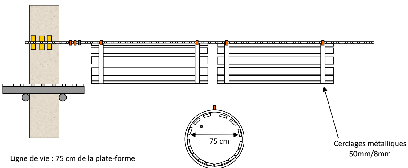
Vue coupe
