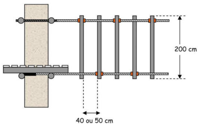
Vue en coupe
