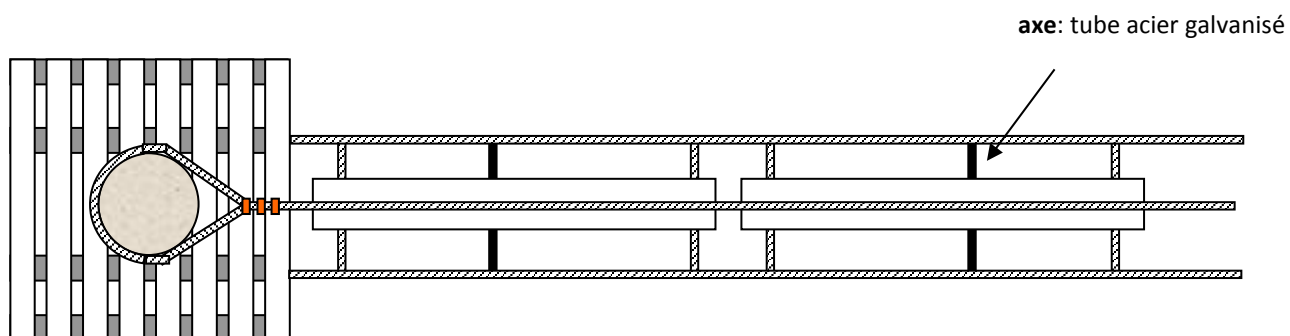
Vue coupe
