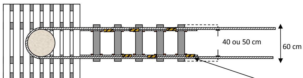
Vue coupe
