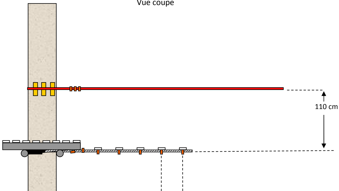
Vue coupe
