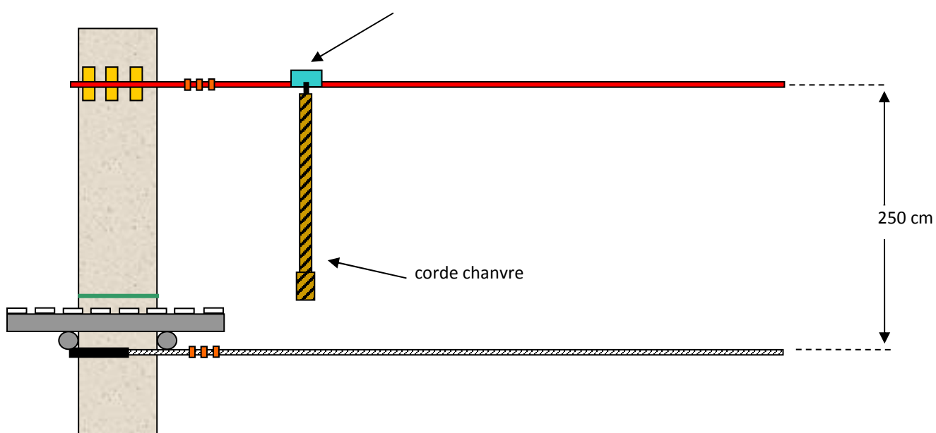
Vue coupe
