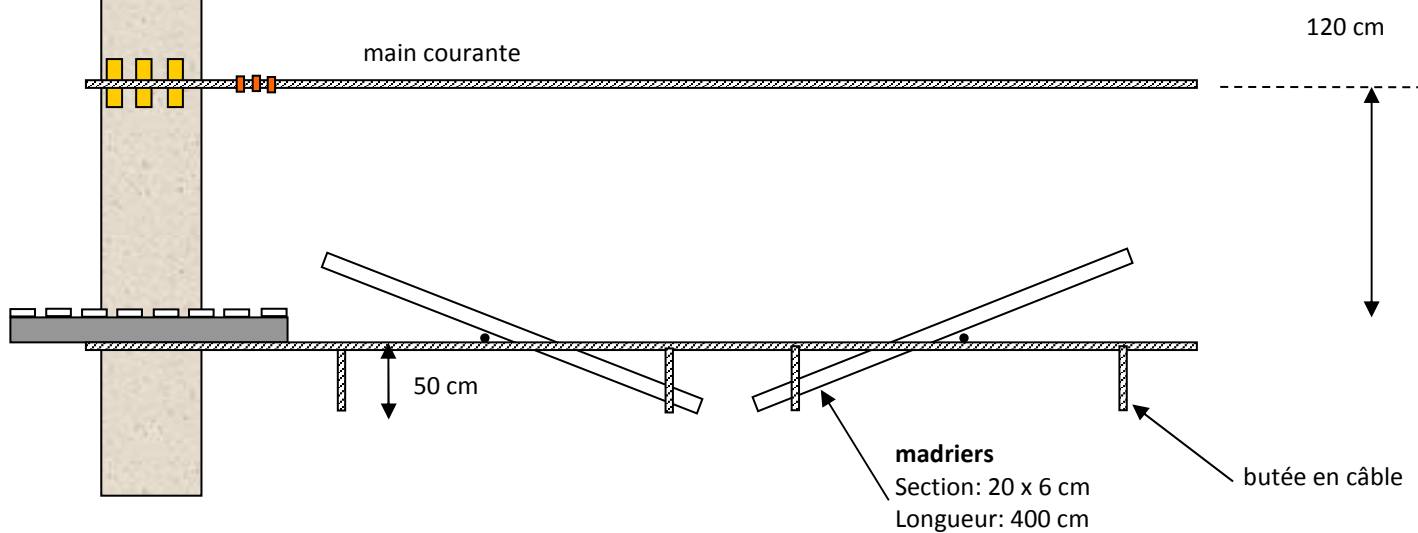
Vue coupe
