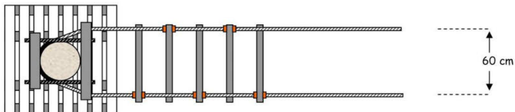
Vue en coupe
